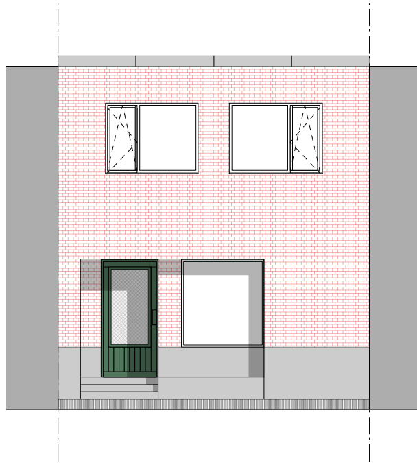
Gevelaanzicht straat
