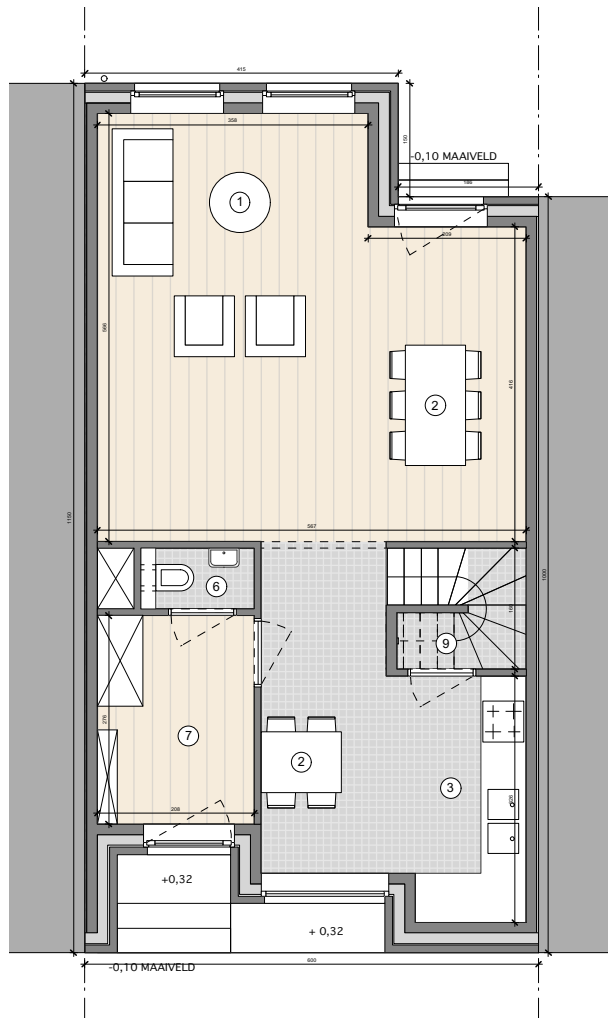
Grondplan niveau 0
