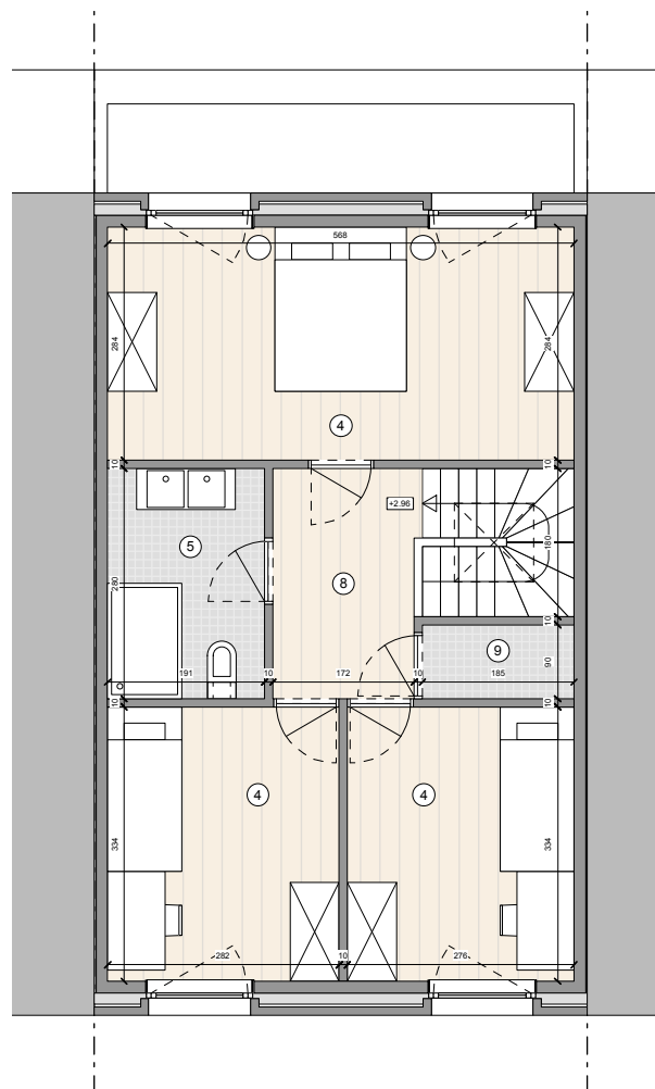
Grondplan niveau +1
