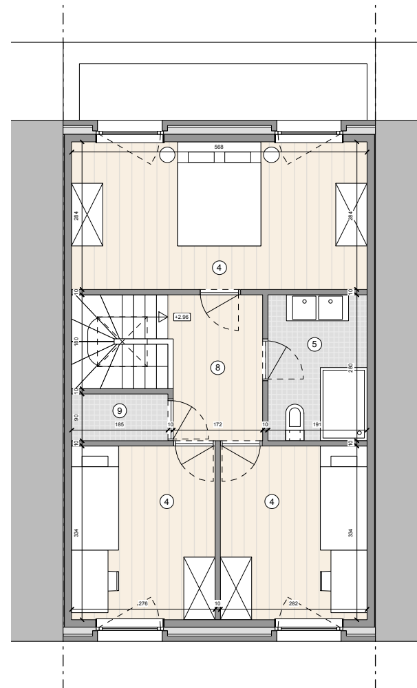
Grondplan niveau +1
