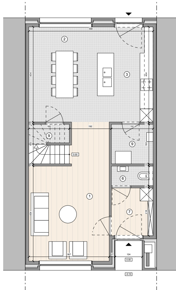
Grondplan niveau 0
