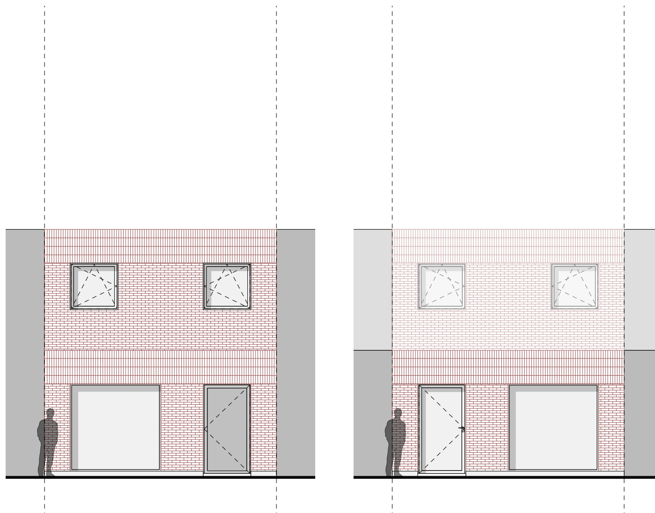
Gevelaanzicht straat
